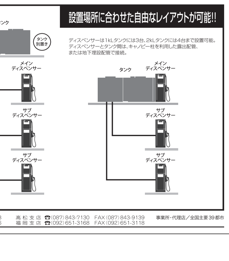
タンク 設置場所に合わせた自由なレイアウトが可能!!
